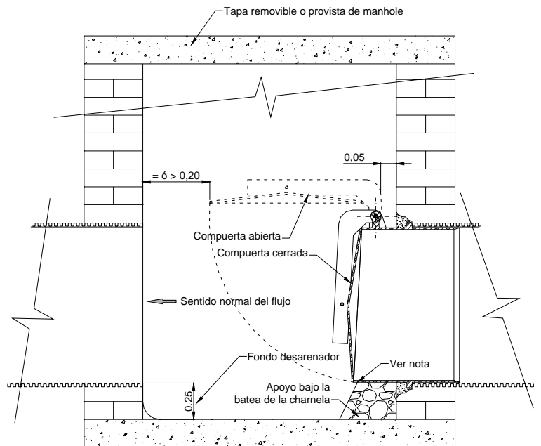
CORTE LONGITUDINAL
